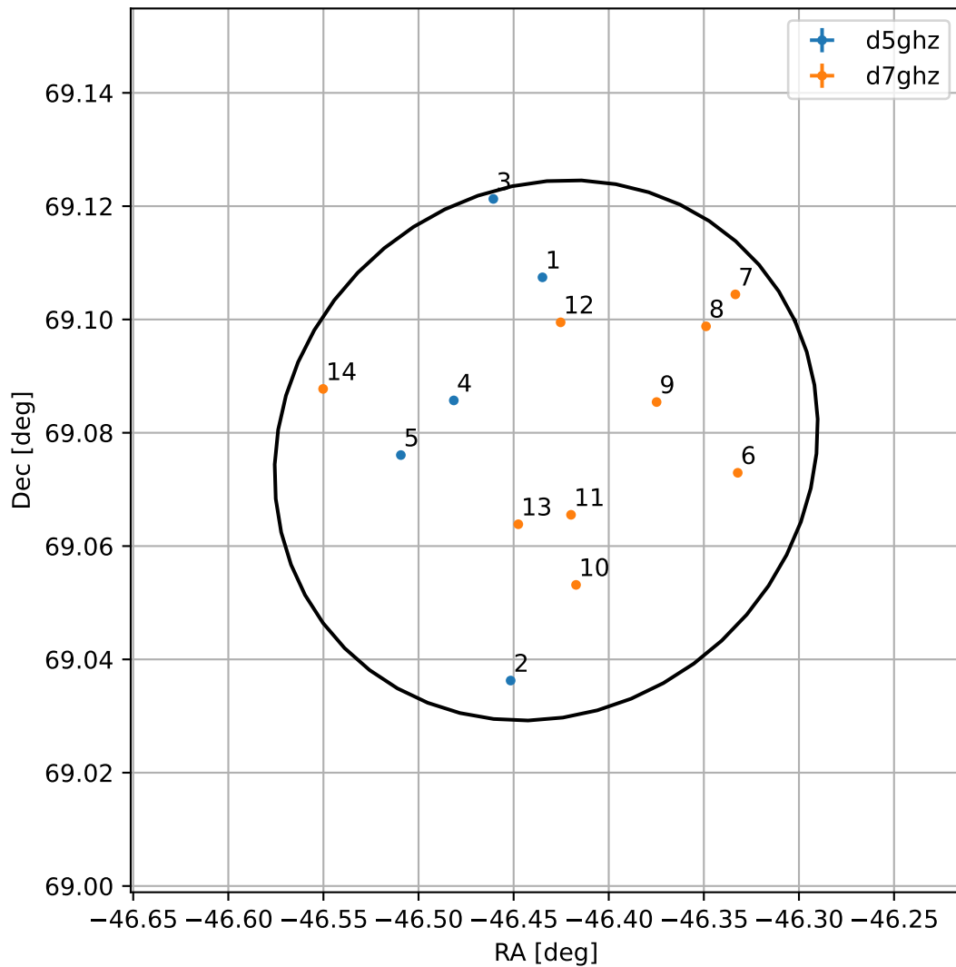
4FGL J2054.2+6904
