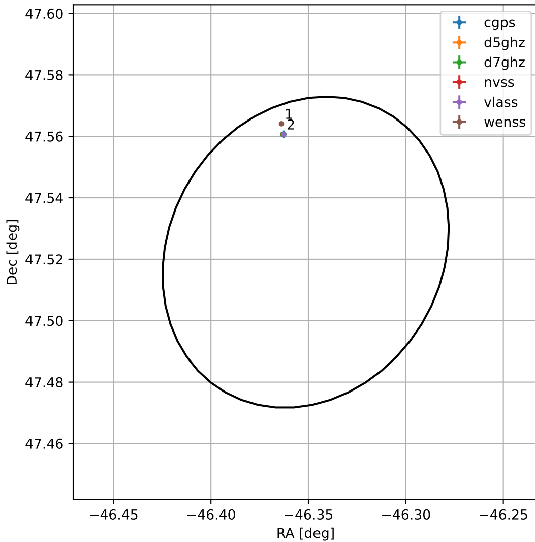
4FGL J2054.5+4731
