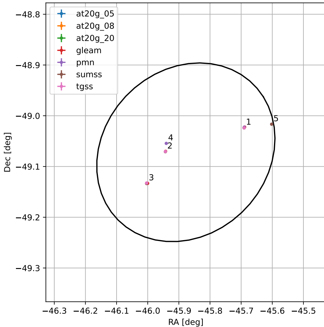
4FGL J2056.4-4904
