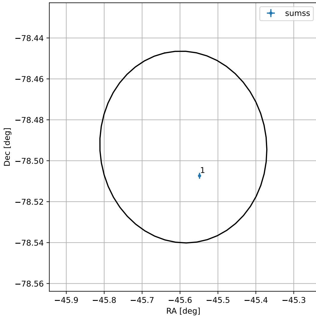
4FGL J2057.6-7829
