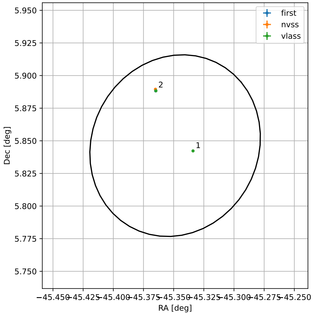
4FGL J2058.6+0550
