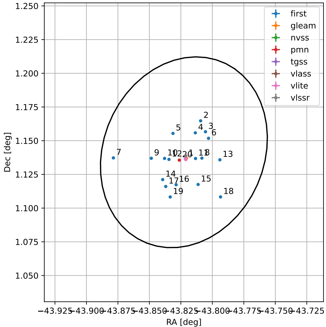
4FGL J2104.7+0108
