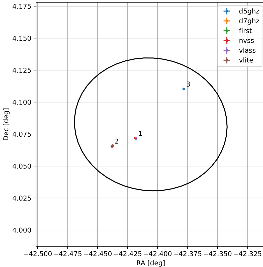
4FGL J2110.3+0404
