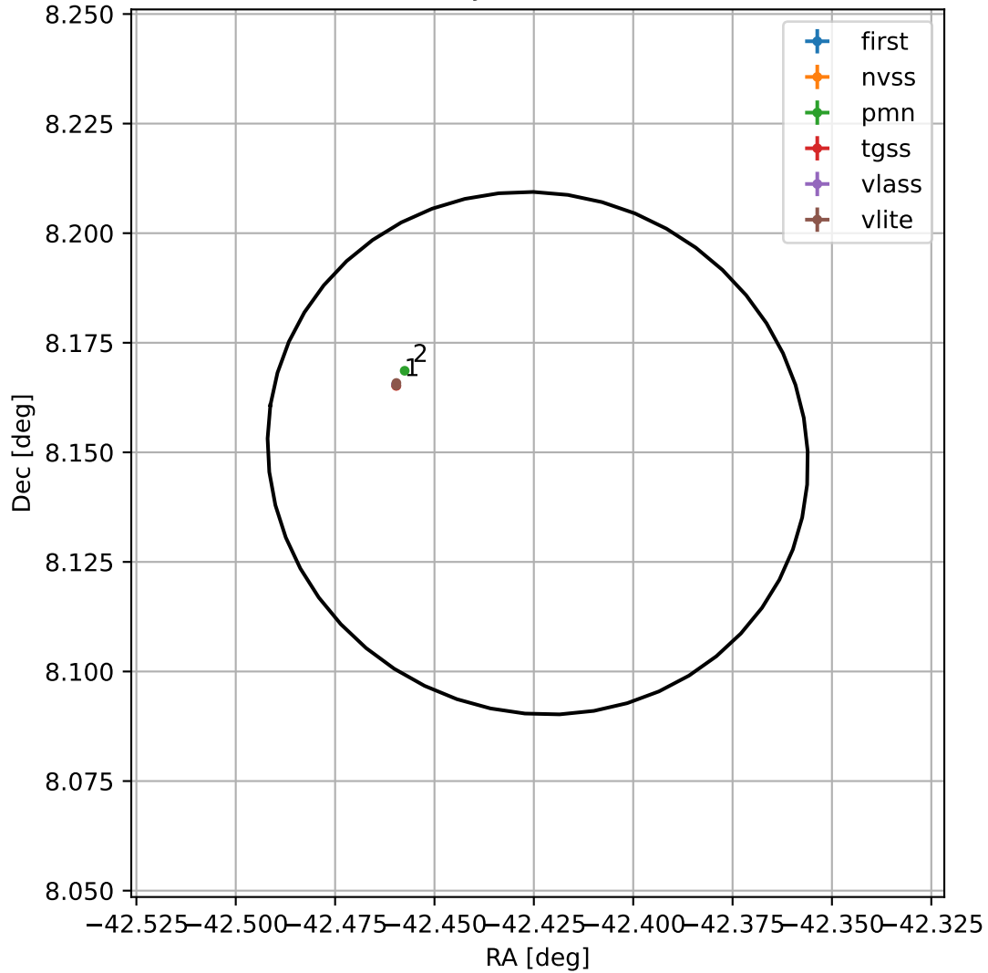
4FGL J2110.3+0808
