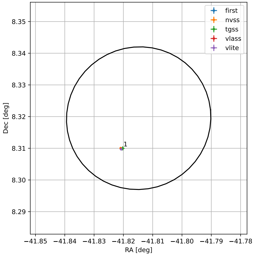
4FGL J2112.7+0819
