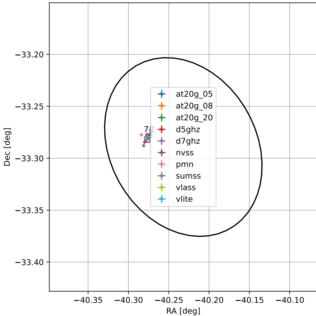
4FGL J2119.0-3317
