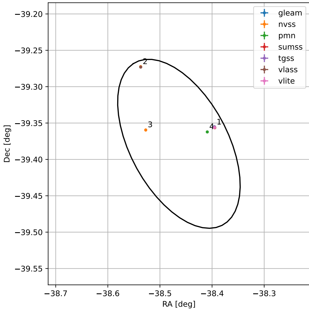
4FGL J2126.1-3922
