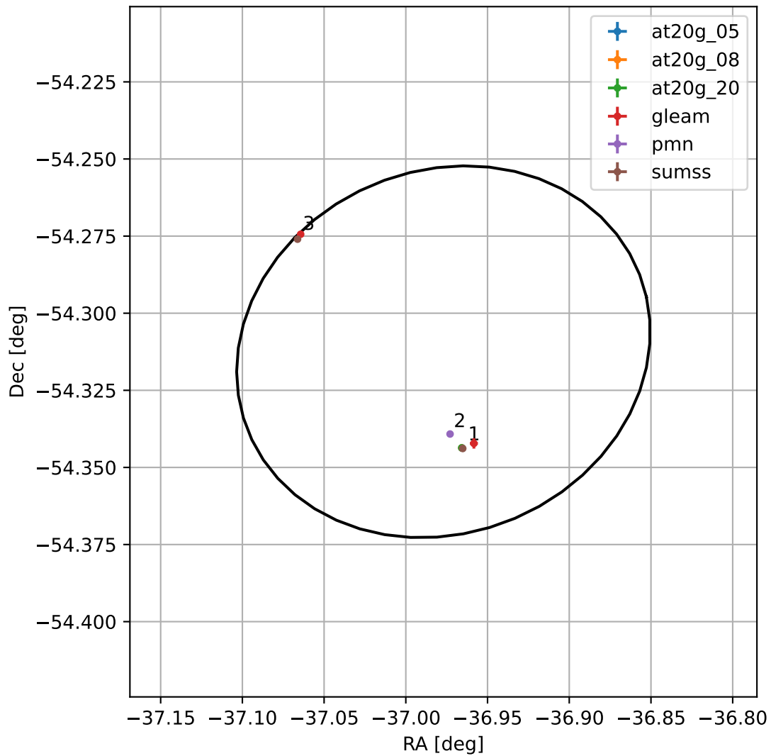
4FGL J2132.0-5418
