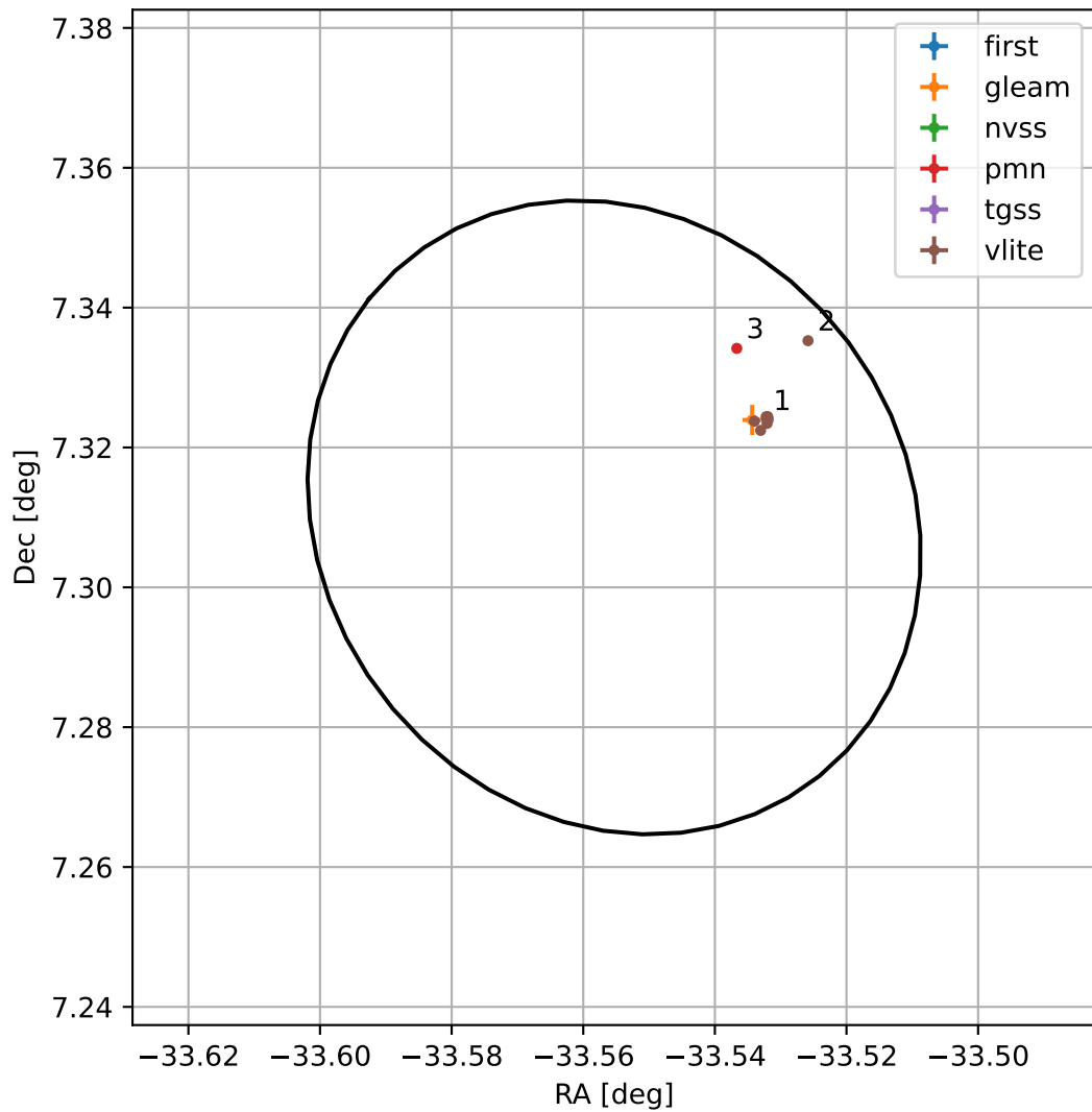
4FGL J2145.7+0718
