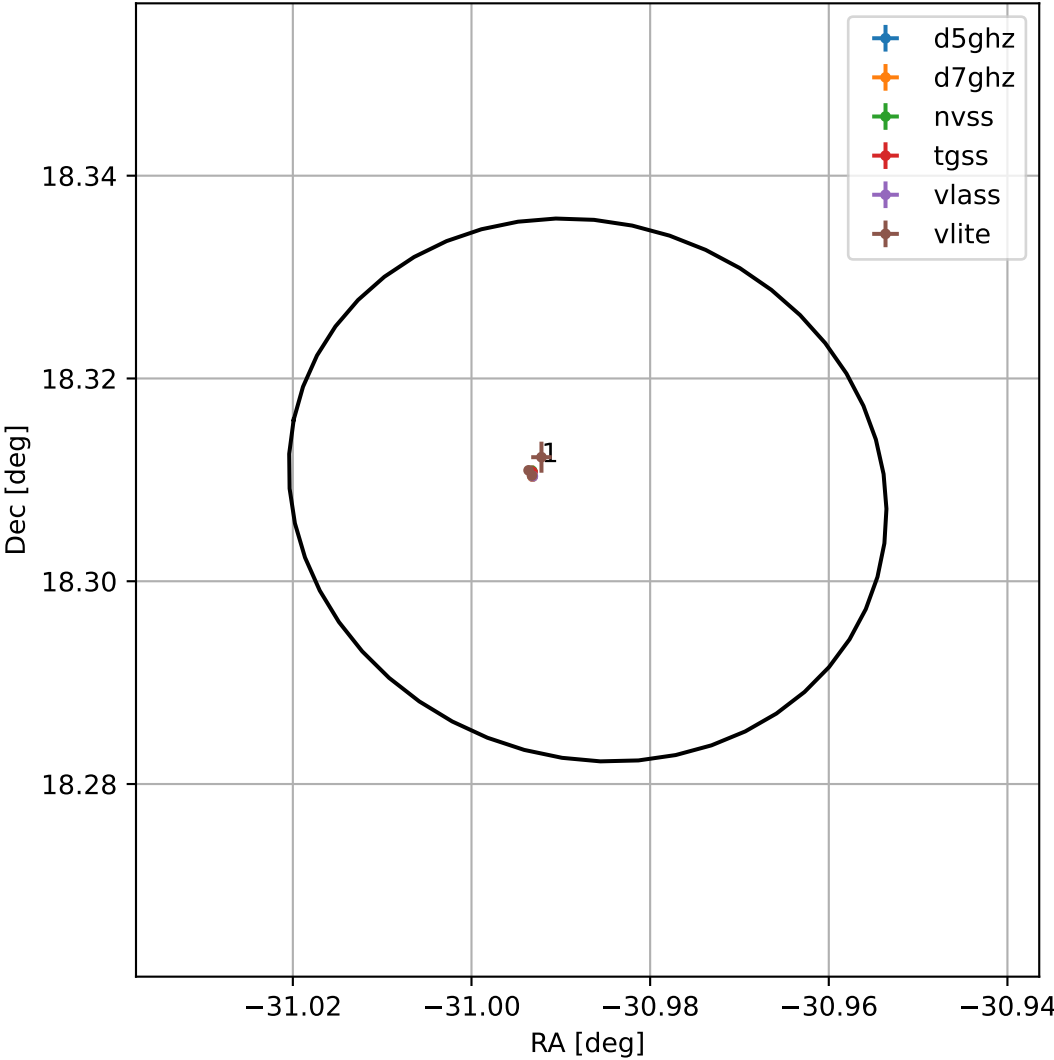
4FGL J2156.0+1818
