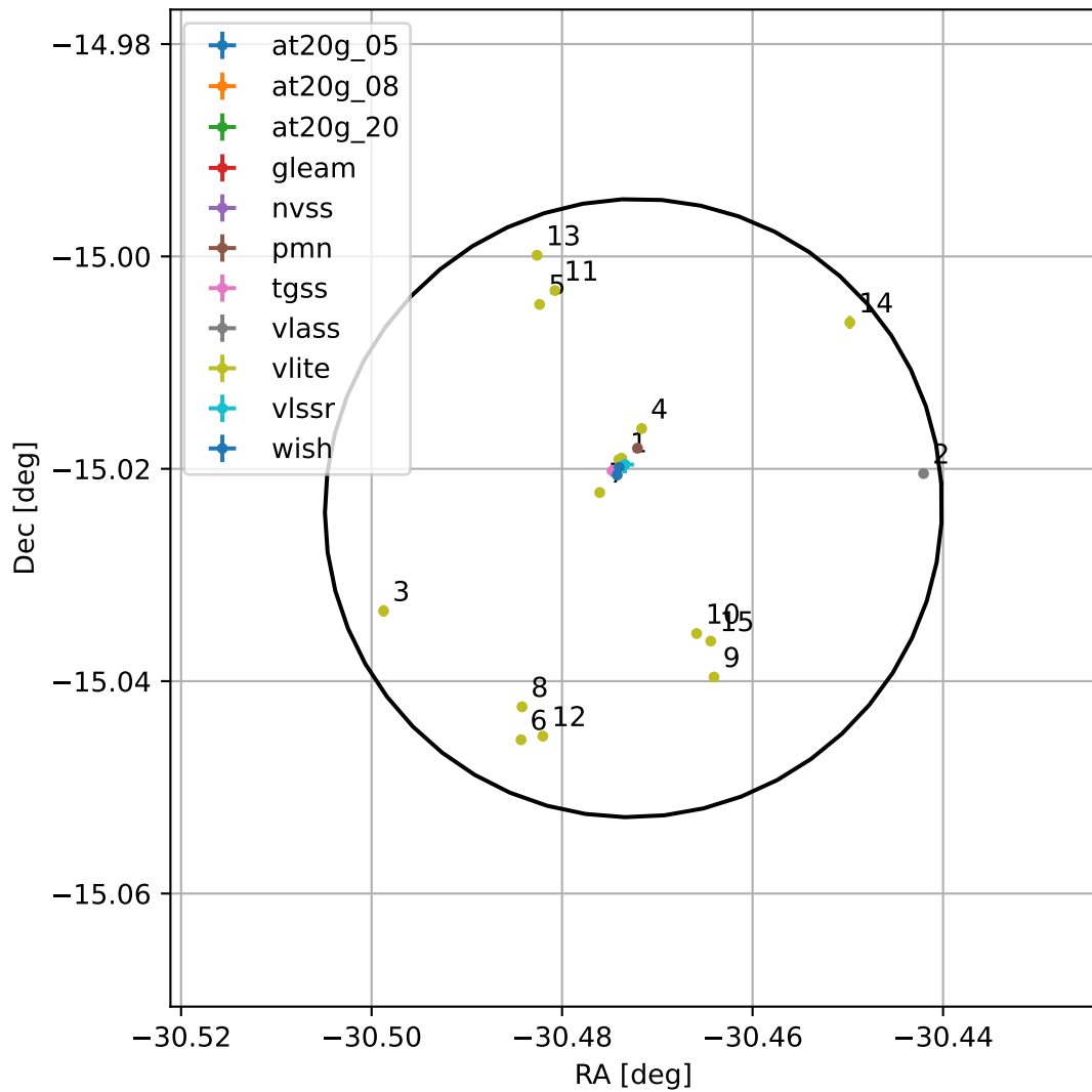
4FGL J2158.1-1501
