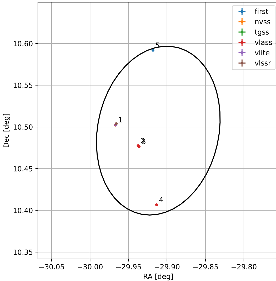
4FGL J2200.3+1029
