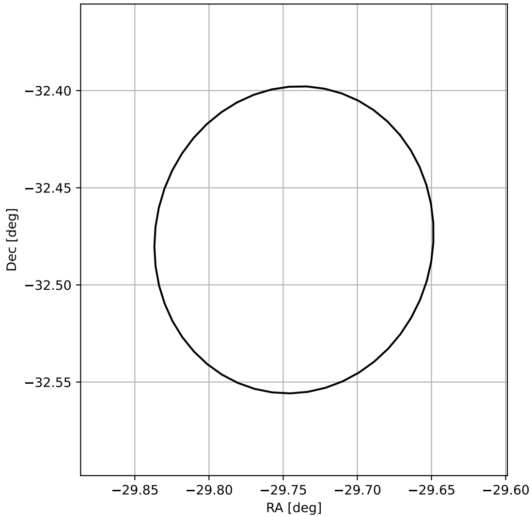
4FGL J2201.0-3228
