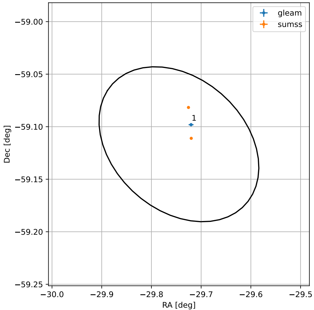
4FGL J2201.0-5907
