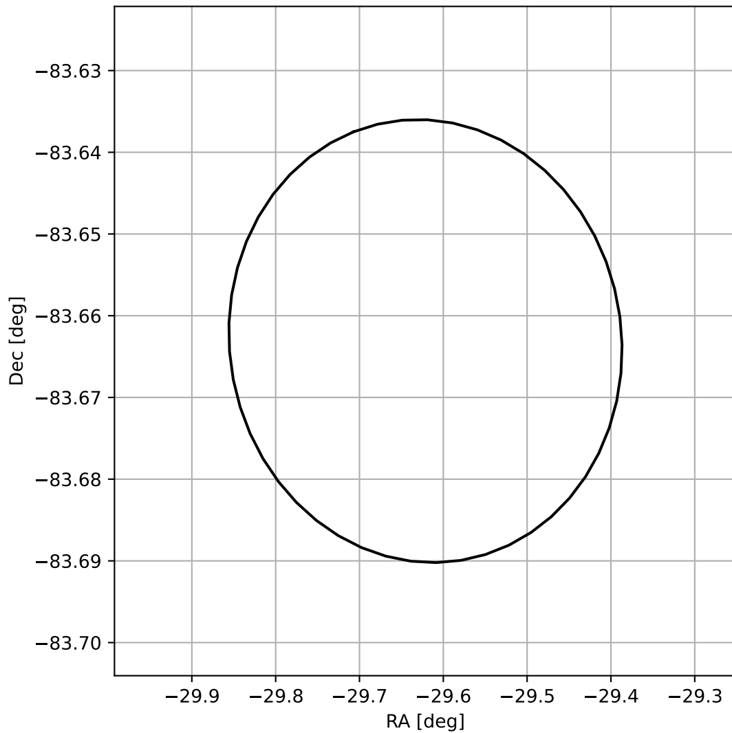
4FGL J2201.5-8339
