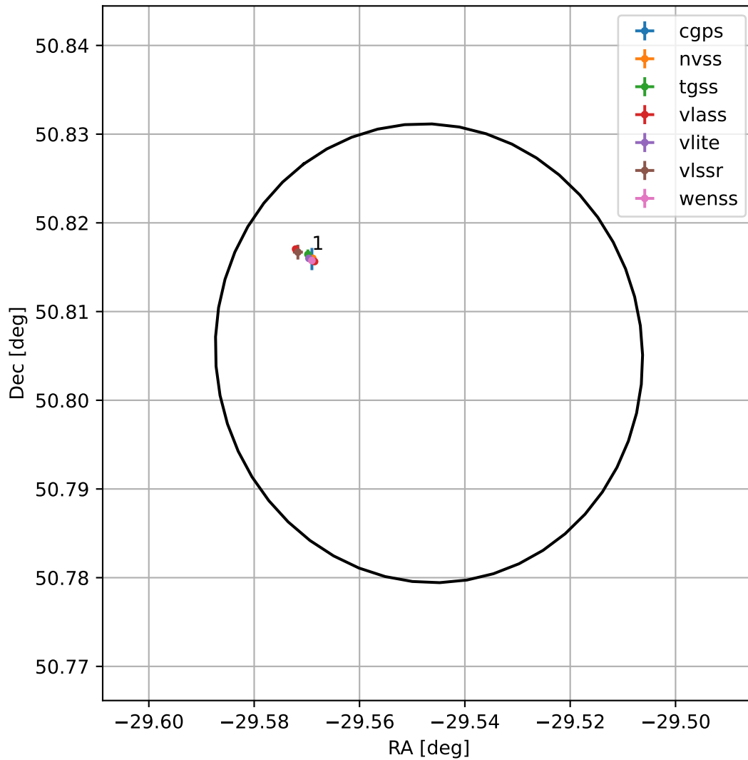
4FGL J2201.8+5048
