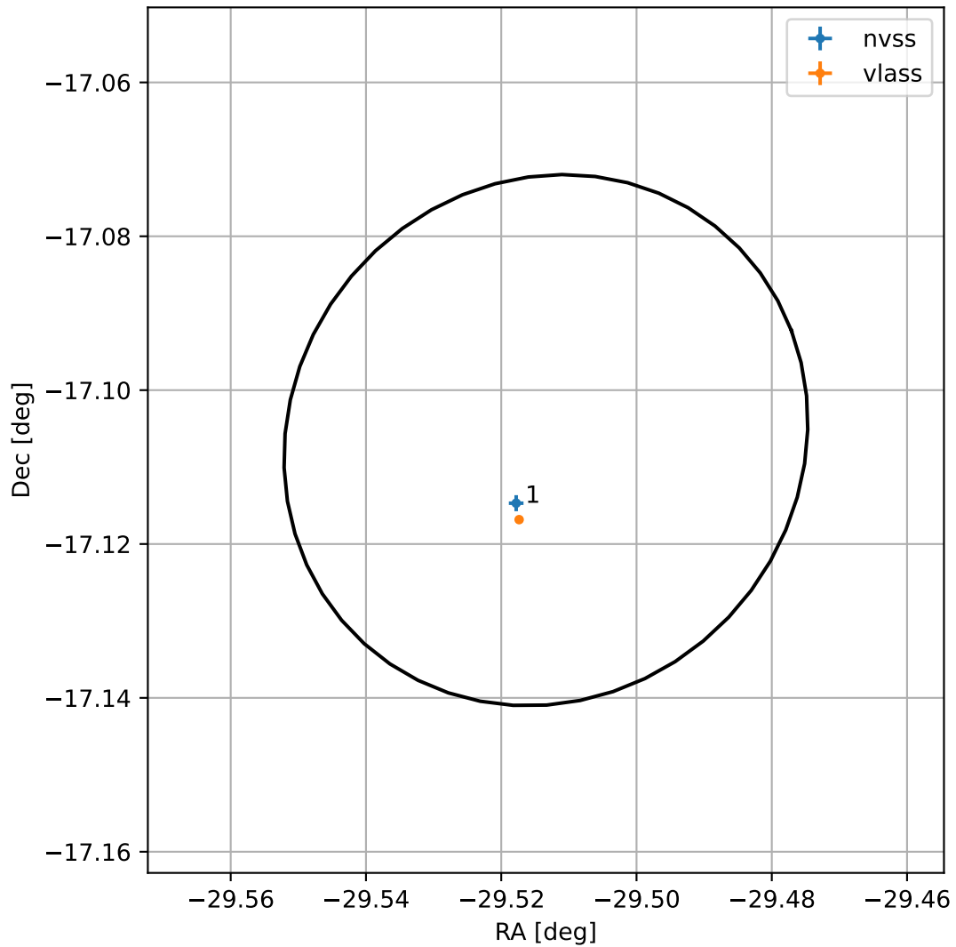
4FGL J2201.9-1706
