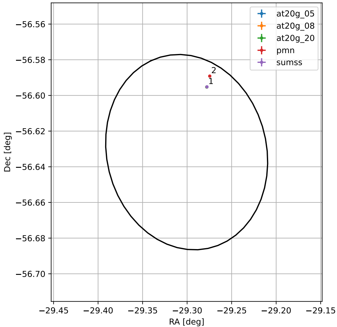
4FGL J2202.7-5637
