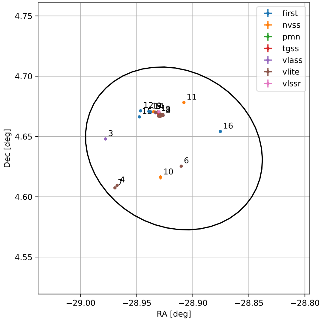
4FGL J2204.3+0438
