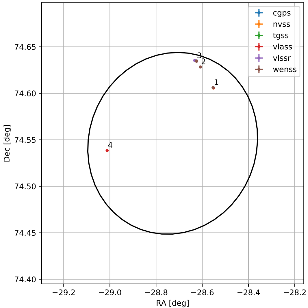
4FGL J2205.0+7432
