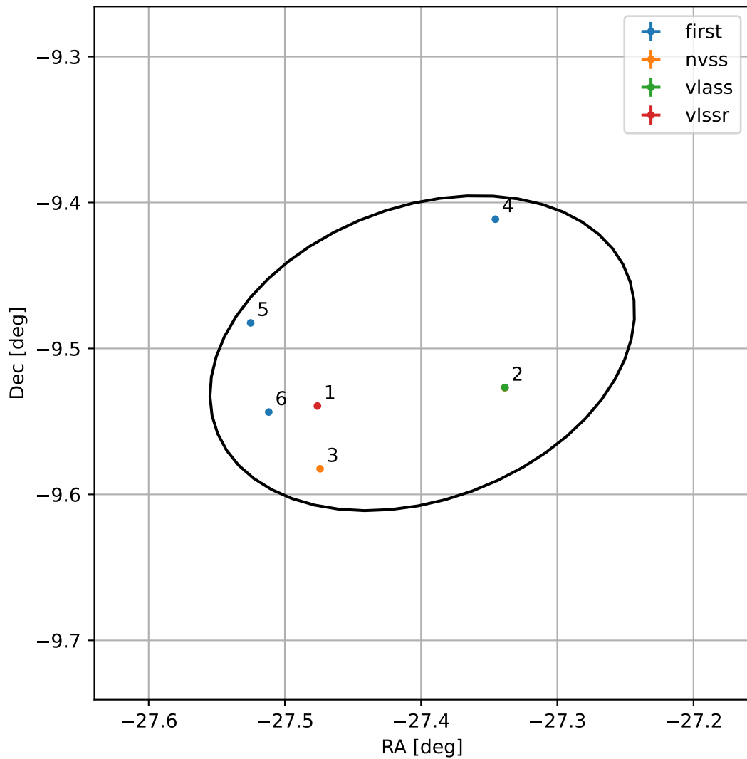
4FGL J2210.4-0930
