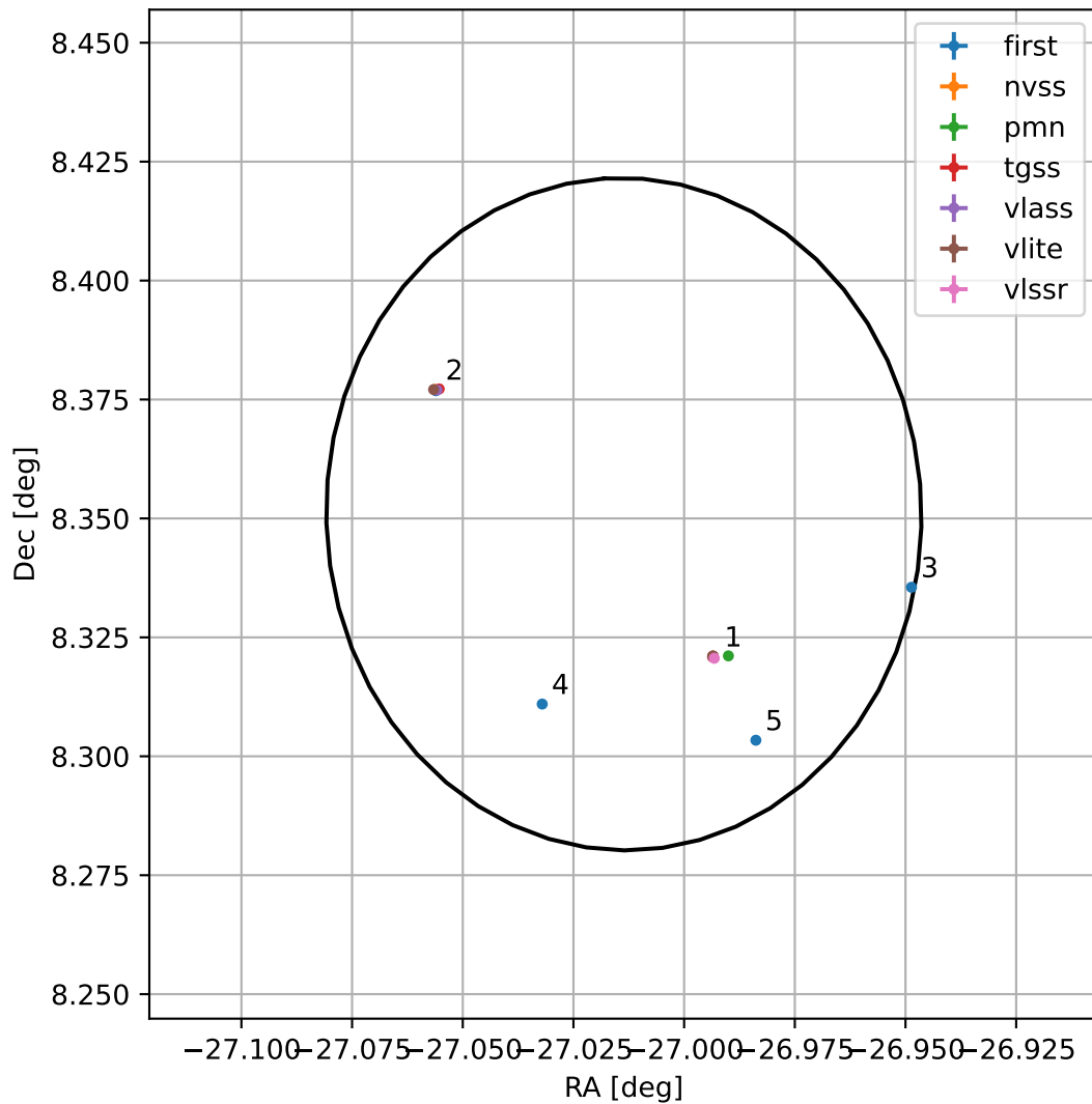
4FGL J2211.9+0821
