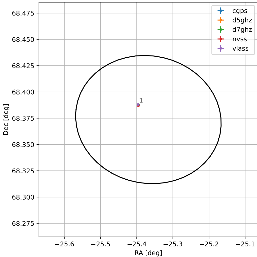
4FGL J2218.5+6822
