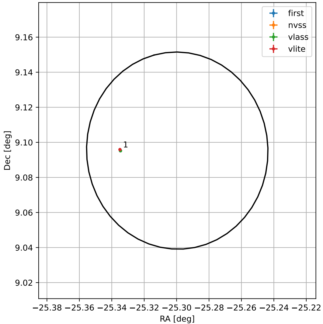
4FGL J2218.8+0905
