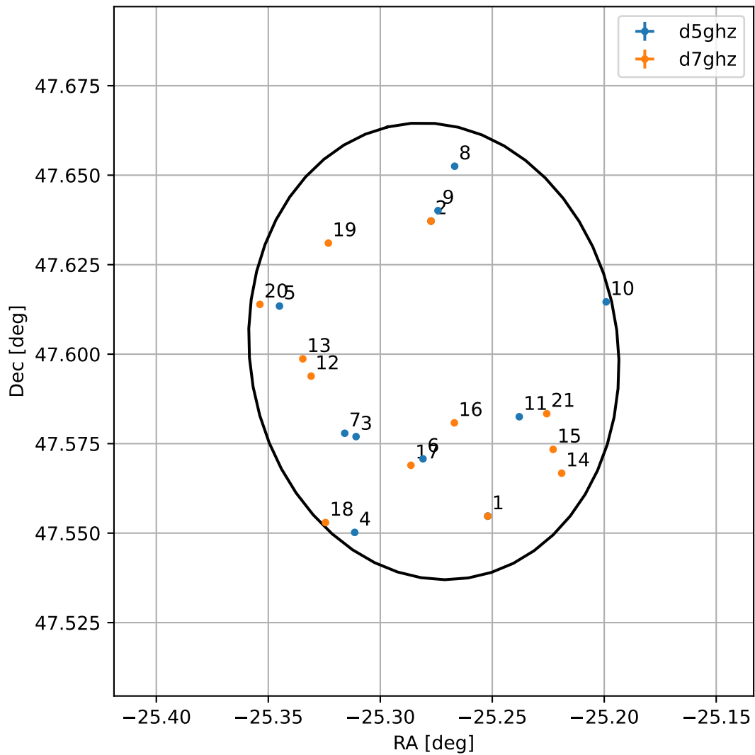
4FGL J2218.8+4736
