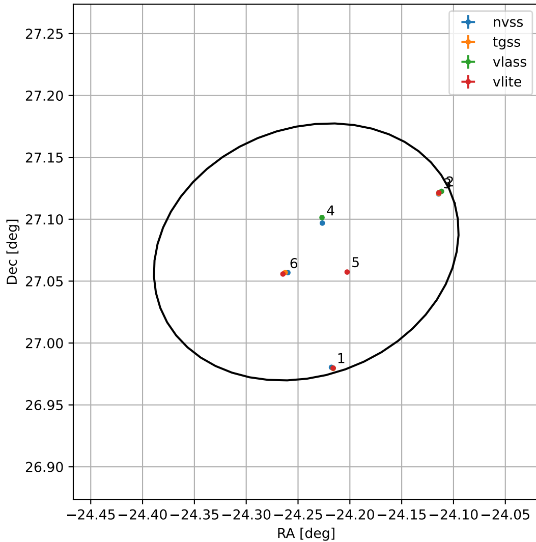
4FGL J2223.0+2704
