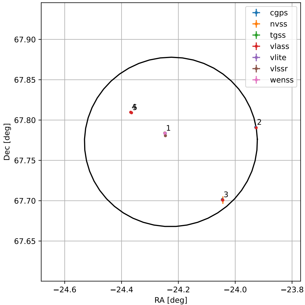
4FGL J2223.0+6746
