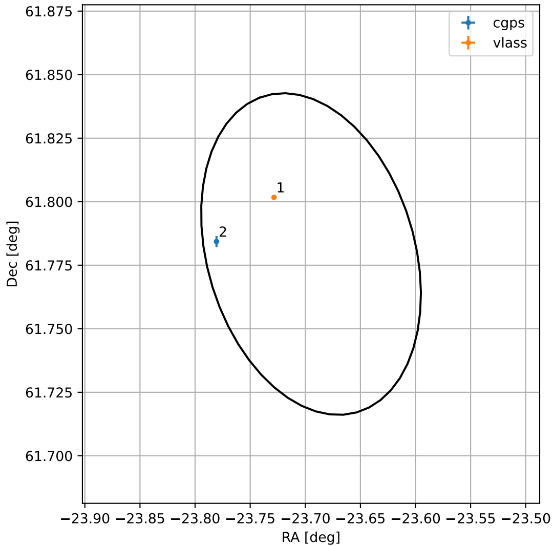
4FGL J2225.2+6146
