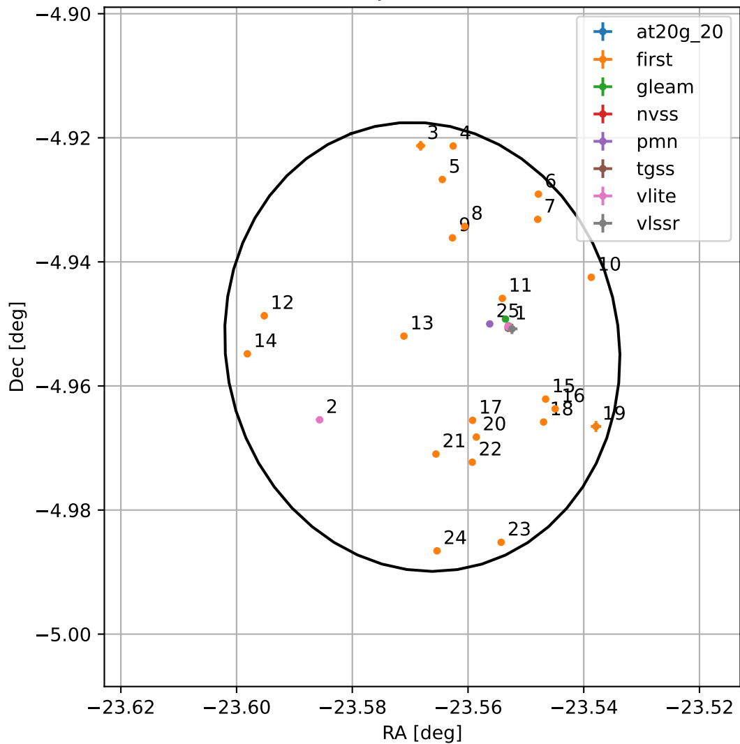
4FGL J2225.7-0457
