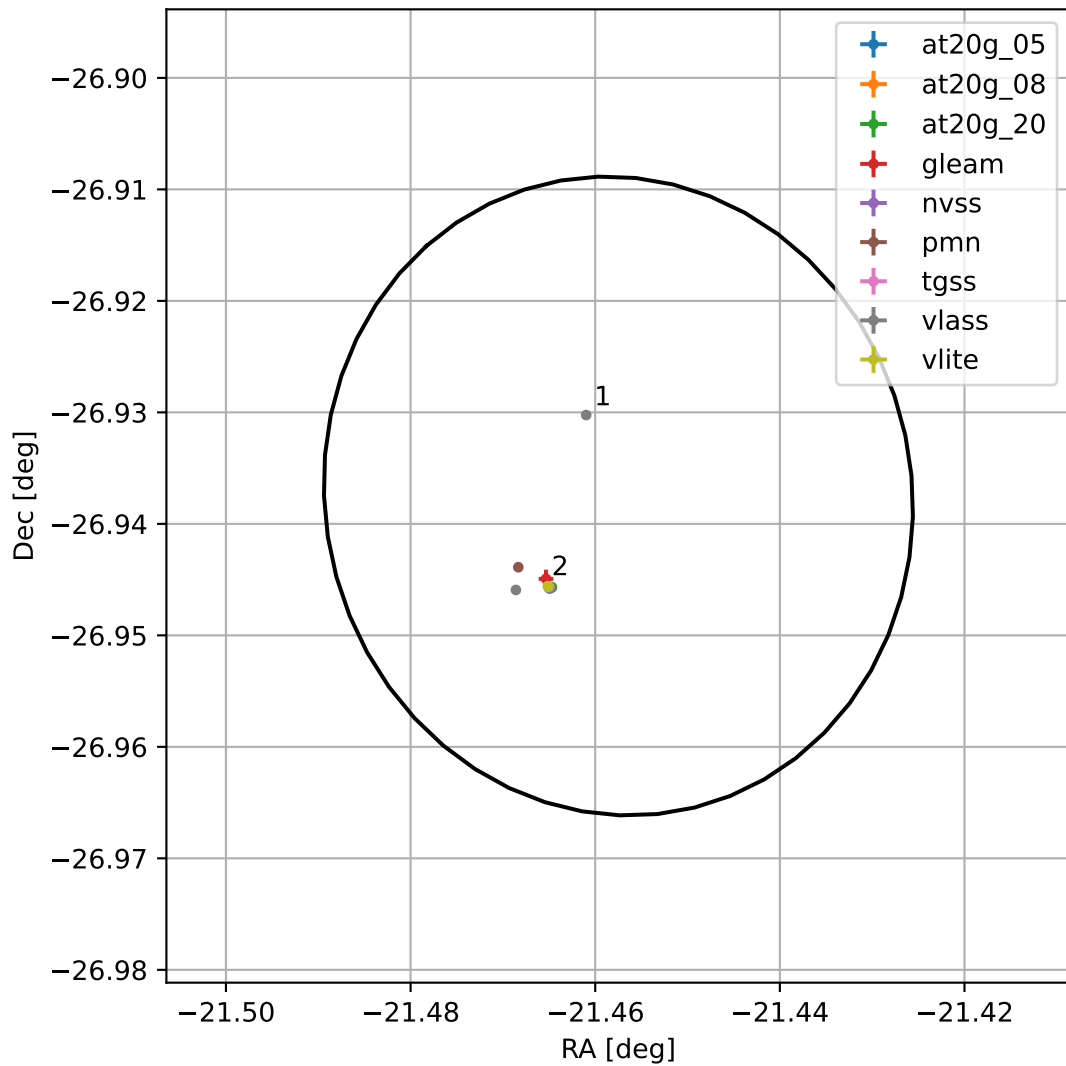
4FGL J2234.1-2656
