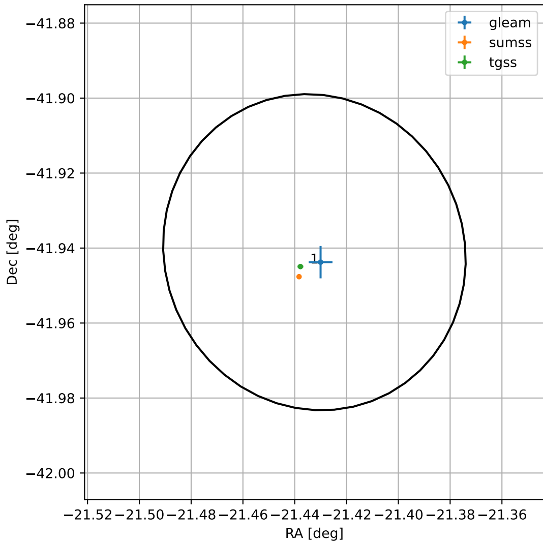
4FGL J2234.2-4156
