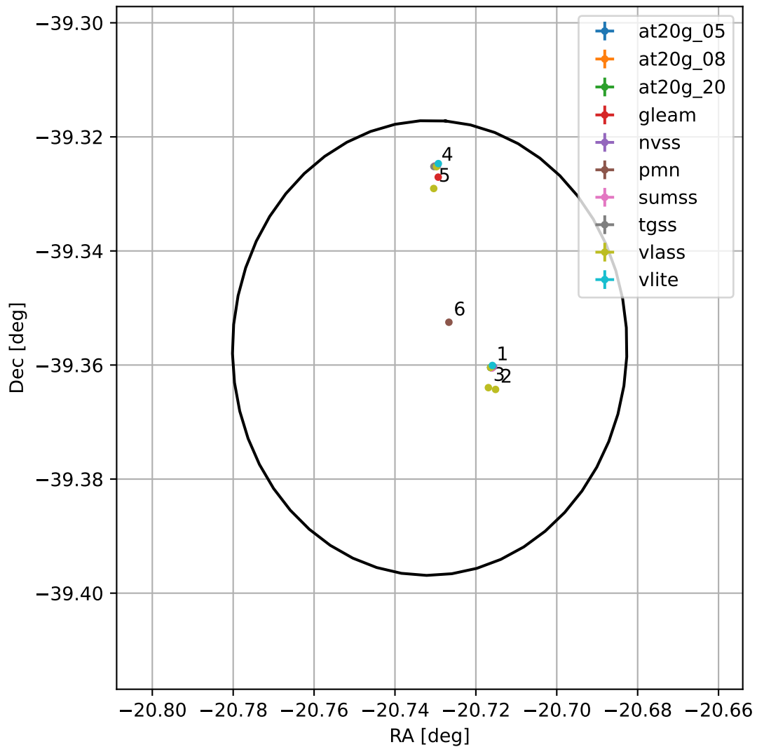
4FGL J2237.0-3921
