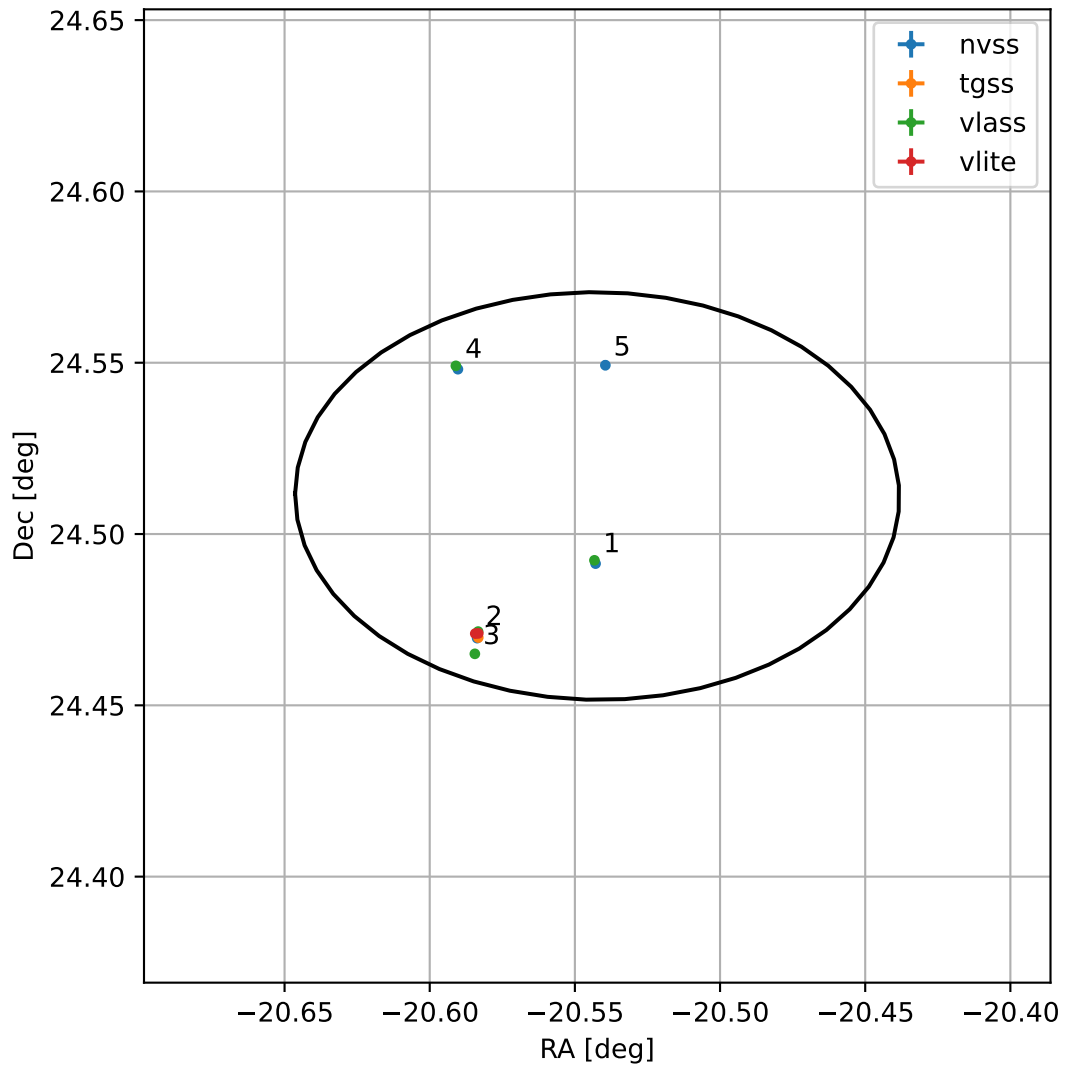
4FGL J2237.8+2430
