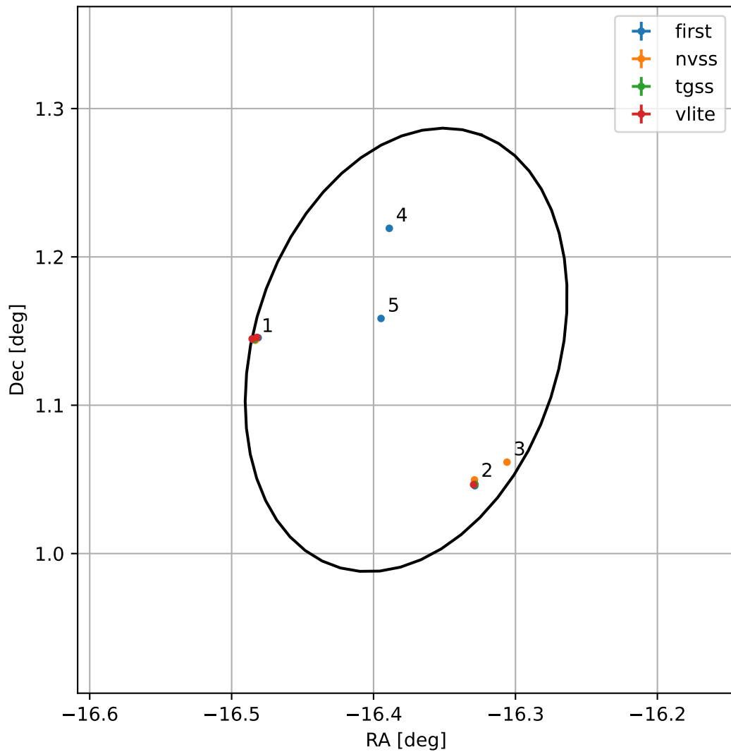
4FGL J2254.4+0108
