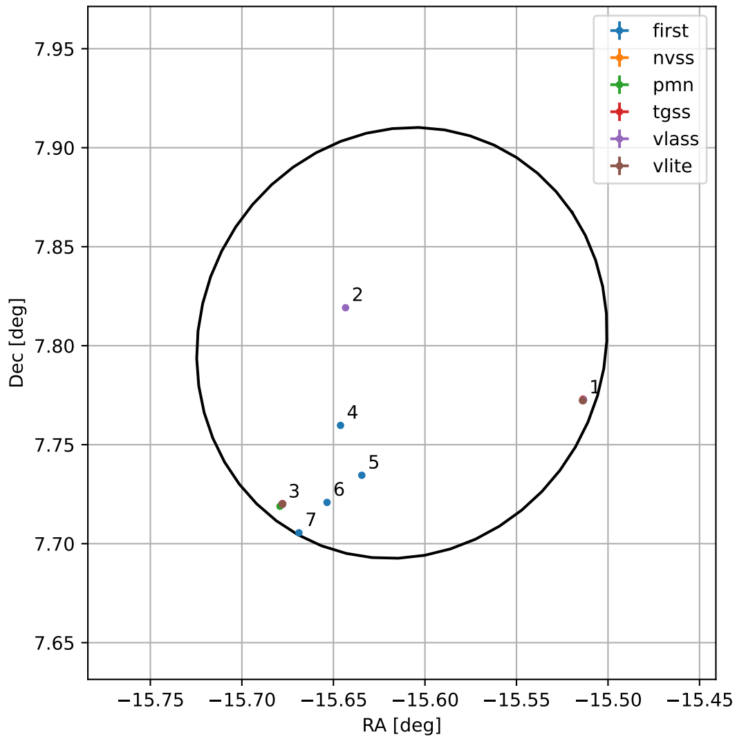
4FGL J2257.5+0748
