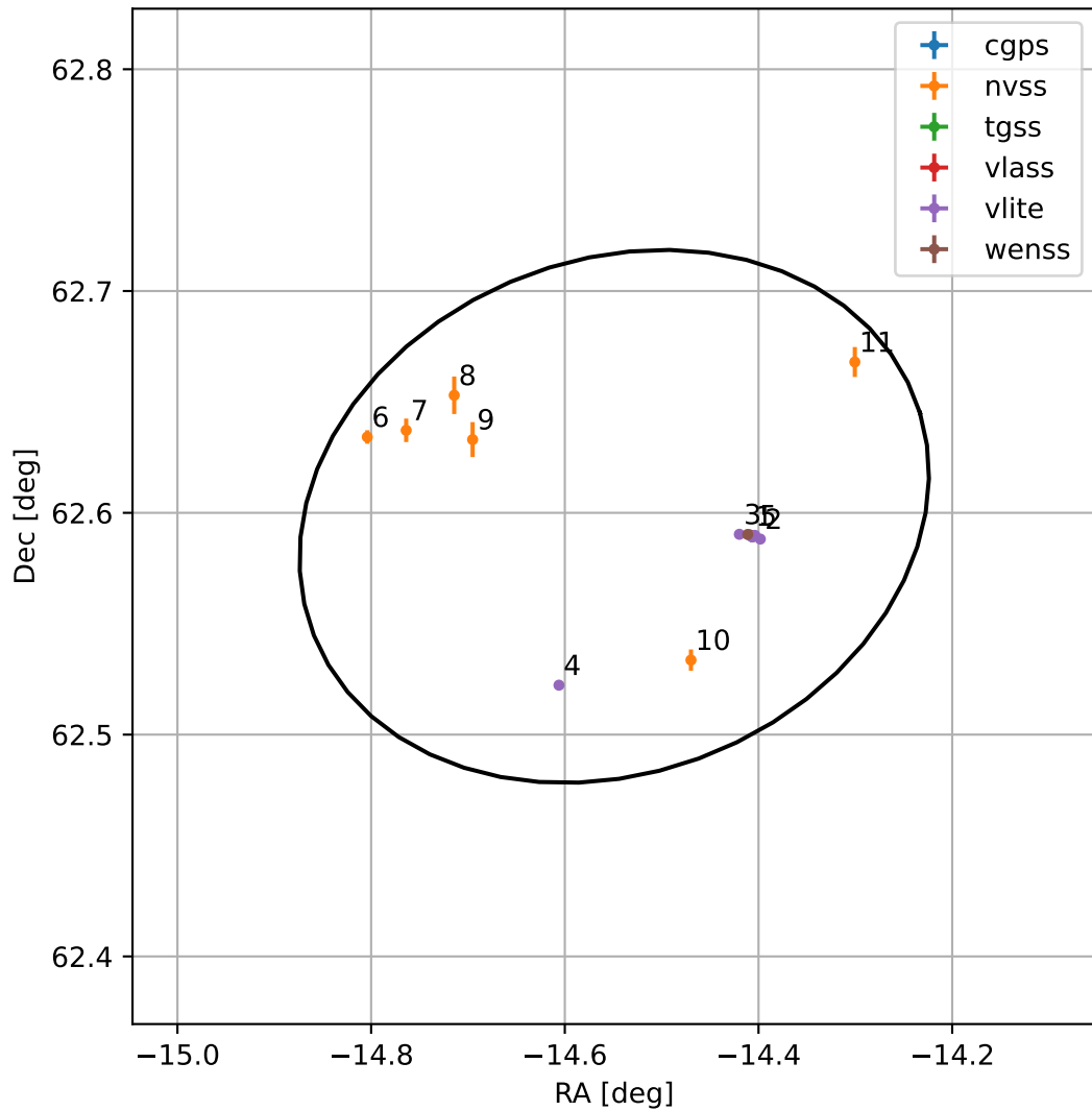
4FGL J2301.8+6235
