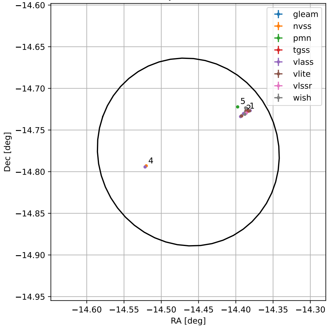
4FGL J2302.1-1446
