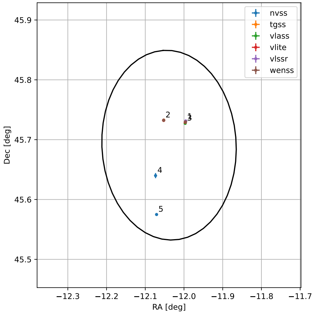
4FGL J2311.8+4541
