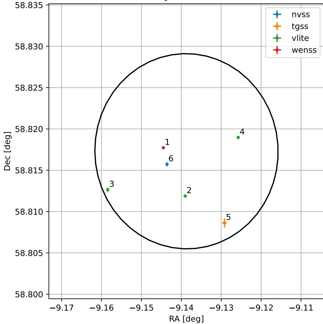
4FGL J2323.4+5849
