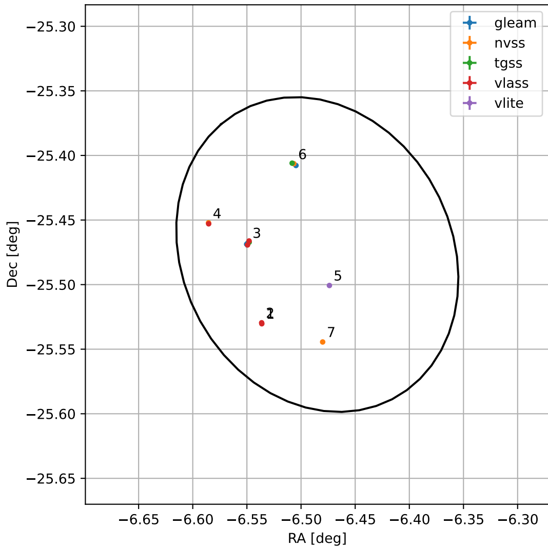
4FGL J2334.0-2528
