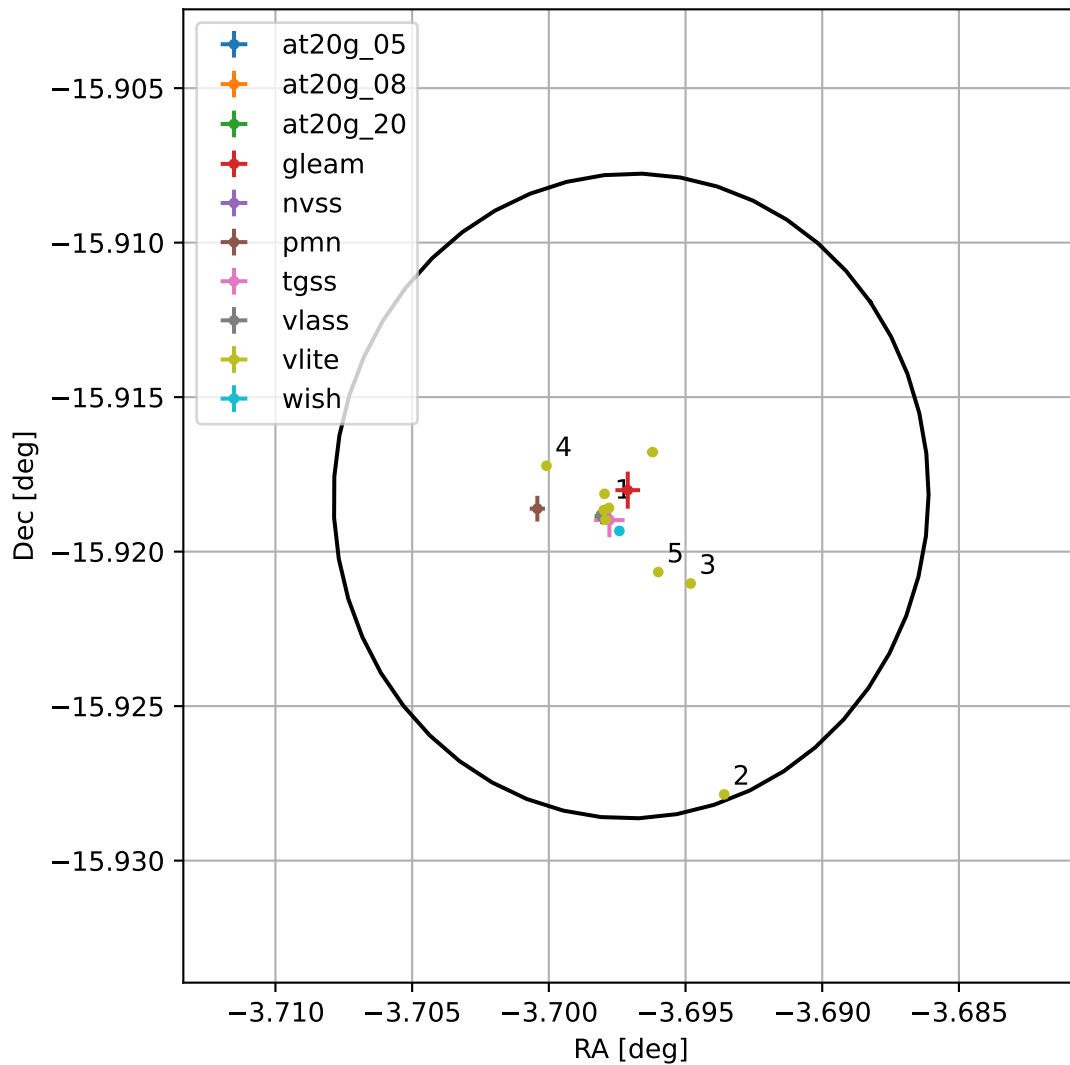
4FGL J2345.2-1555
