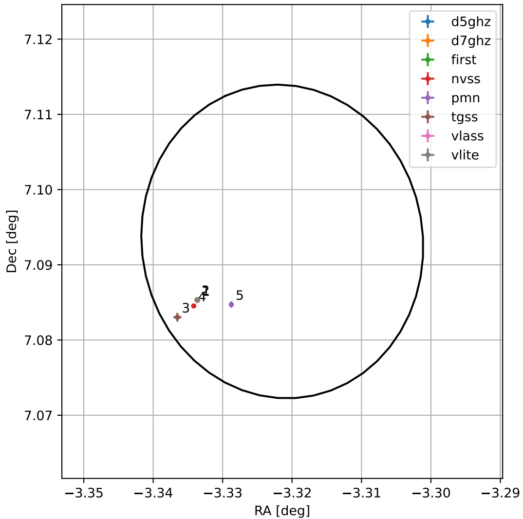
4FGL J2346.7+0705
