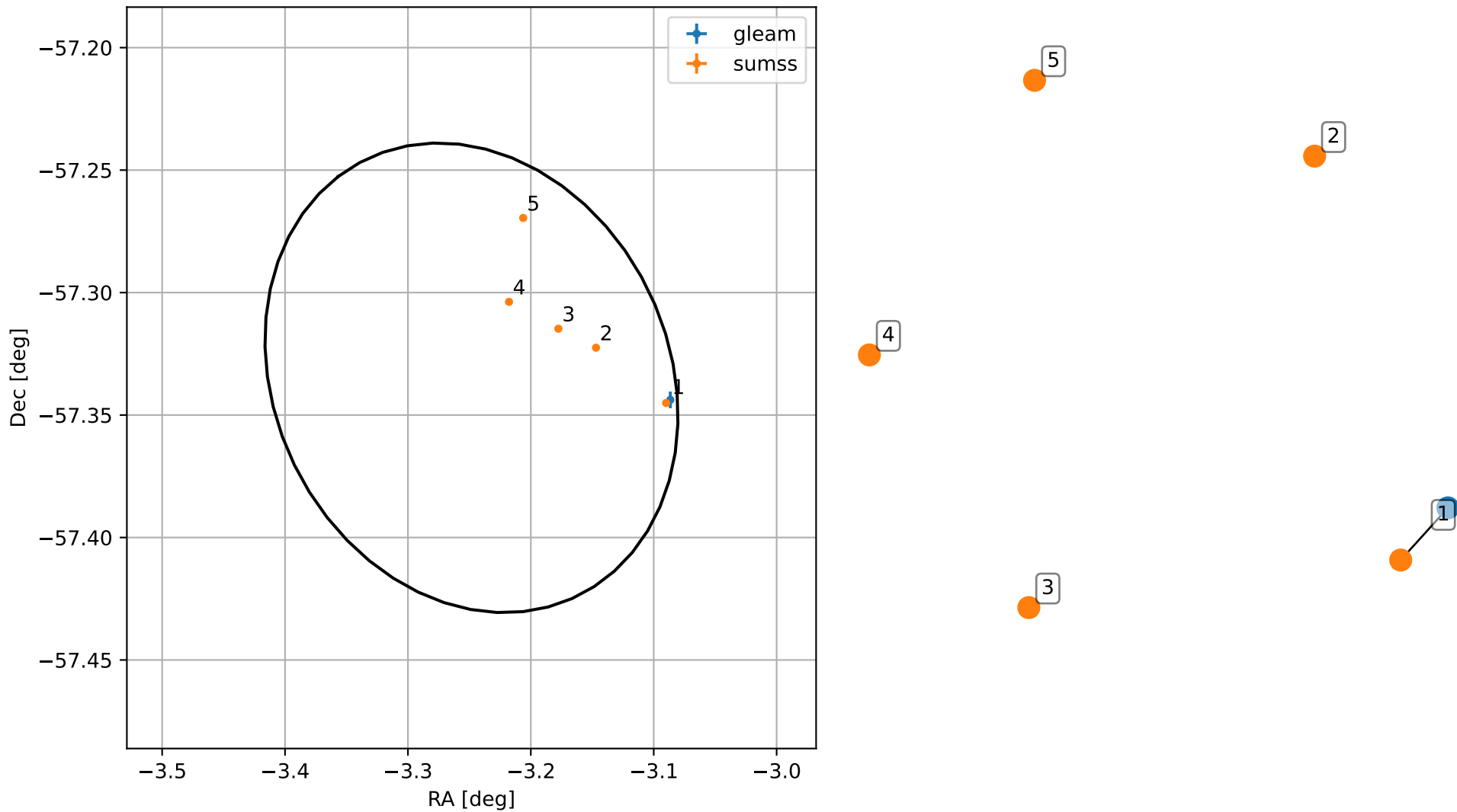
4FGL J2347.0-5720
