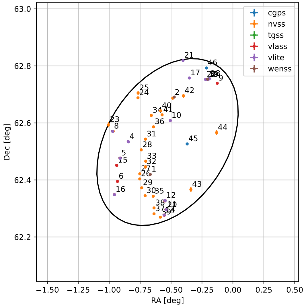
4FGL J2357.8+6231
