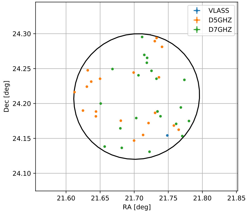
4FGL J0126.8+2412
