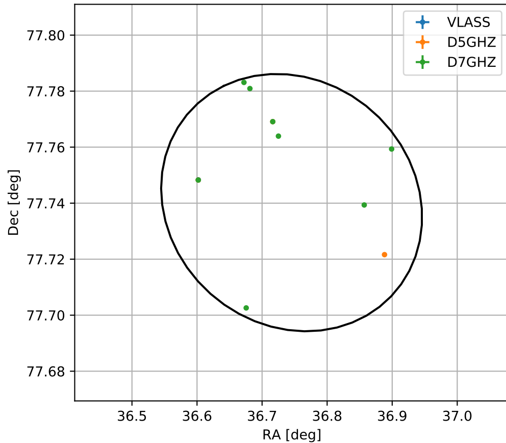
4FGL J0226.9+7744
